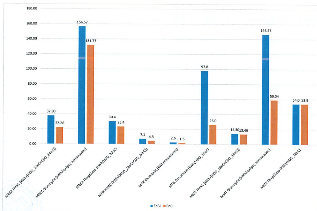
Σχήμα 19: Σύγκριση κανονικοποιημένων δεικτών ενεργειακής απόδοσης (EnPI) για το 2022 με δείκτες γραμμής βάσης (EnBI).
