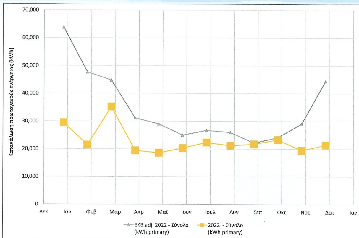
Σχήμα 13: Μηνιαία κατανάλωση πρωτογενούς ενέργειας (kWh) έτους 2022 στο ΜΠΚ συγκριτικά με EKB ± προσαρμογές (EKB ± adj. 2021).
