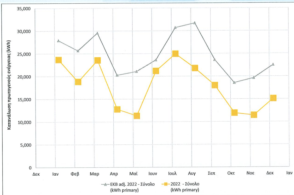
Σχήμα 17: Μηνιαία κατανάλωση πρωτογενούς ενέργειας (kWh) έτους 2022 στο ΜΜΤ συγκριτικά με ΕΚΒ ± προσαρμογές (ΕΚΒ ± adj. 2022).
