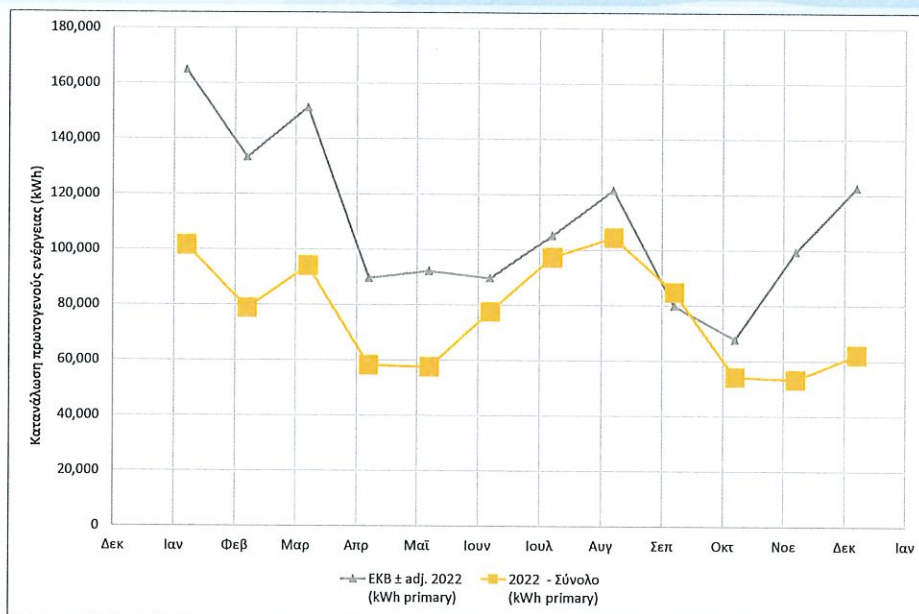
Σχήμα 18: Μηνιαία κατανάλωση πρωτογενούς ενέργειας (kWh) έτους 2022 στα 3 Μουσεία συγκριτικά με ΕΚΒ ± προσαρμογές (ΕΚΒ ± adj. 2022).
