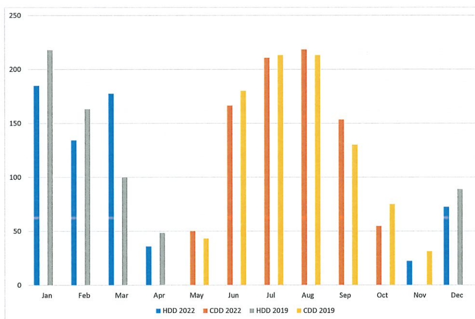
Σχήμα 15: Βαθμοημέρες θέρμανσης (αριστερός άξονας) και ψύξης (δεξιός άξονας) ανά μήνα για το 2022 συγκριτικά με το 2019 στο ΜΜΤ
