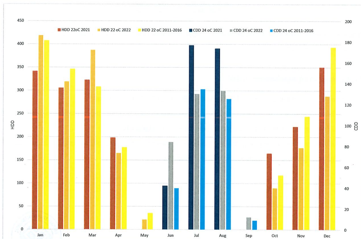
Σχήμα 11: Βαθμοημέρες θέρμανσης (αριστερός άξονας) και ψύξης (δεξιός άξονας) ανά μήνα για το 2022 συγκριτικά με το 2021 και την περίοδο 2011-2016 στο ΜΠΚ
