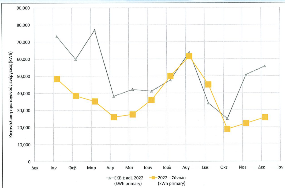
Σχήμα 9: Μηνιαία κατανάλωση πρωτογενούς ενέργειας (kWh) έτους 2022 στο ΜΒΕΛ συγκριτικά με EKB ± προσαρμογές (EKB ± adj. 2022).
