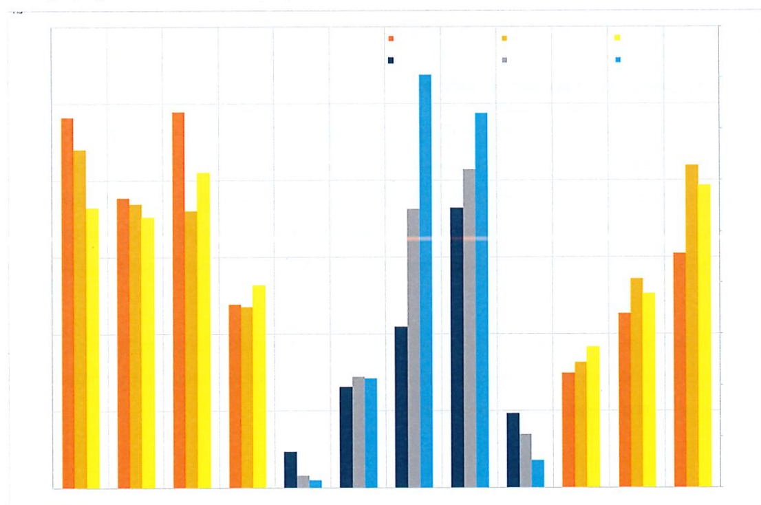
Σχήμα 7: Βαθμοημέρες θέρμανσης (αριστερός άξονας) και ψύξης (δεξιός άξονας) ανά μήνα για το 2022 συγκριτικά με το 2021 και την περίοδο 2011-2016 στο ΜΒΕΛ
