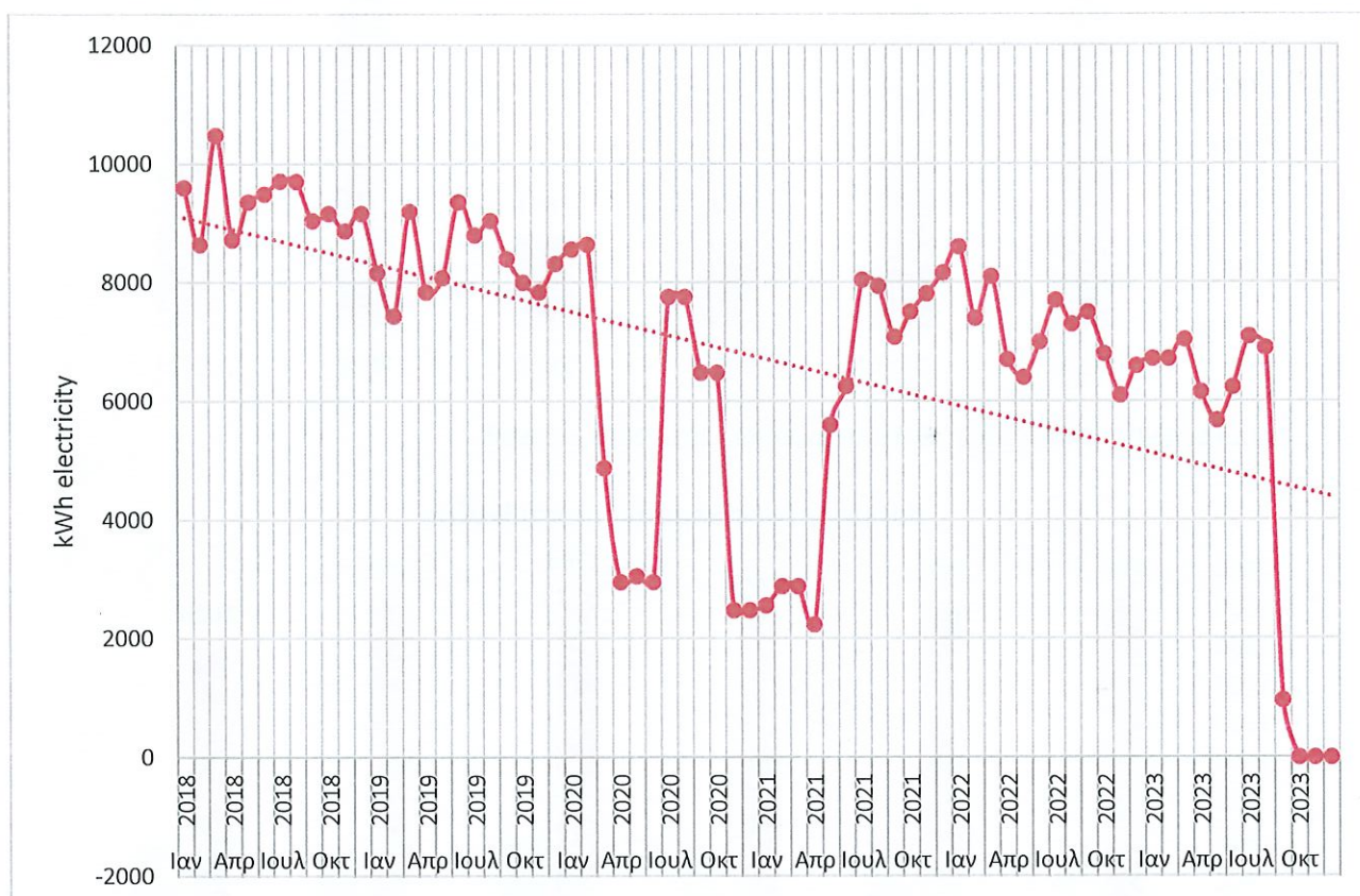
Σχήμα 8: Μηνιαία κατανάλωση ηλεκτρικής ενέργειας σύμφωνα με στοιχεία λογαριασμών ηλεκτρικής ενέργειας περιόδου 2018-2021.
