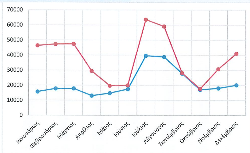
Σχήμα 16: Μηνιαία κατανάλωση πρωτογενούς ενέργειας (kWh) έτους 2023 στο ΜΒΕΛ συγκριτικά με ΕΚΒ ± προσαρμογές (ΕΚΒ ± adj. 2021).
