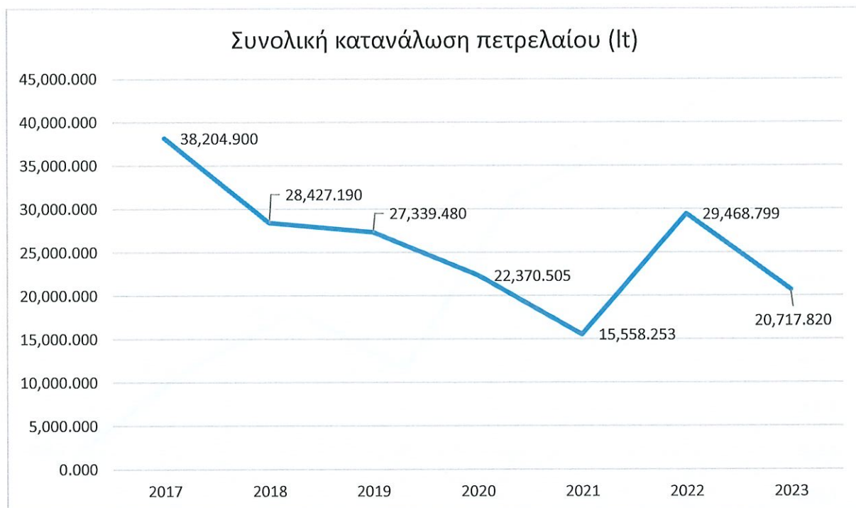
Σχήμα 3: Εξέλιξη ετήσιας κατανάλωσης πετρελαίου θέρμανσης την περίοδο 2017-2023 στο σύνολο των κτηριακών υποδομών του ΠΙΟΠ.
