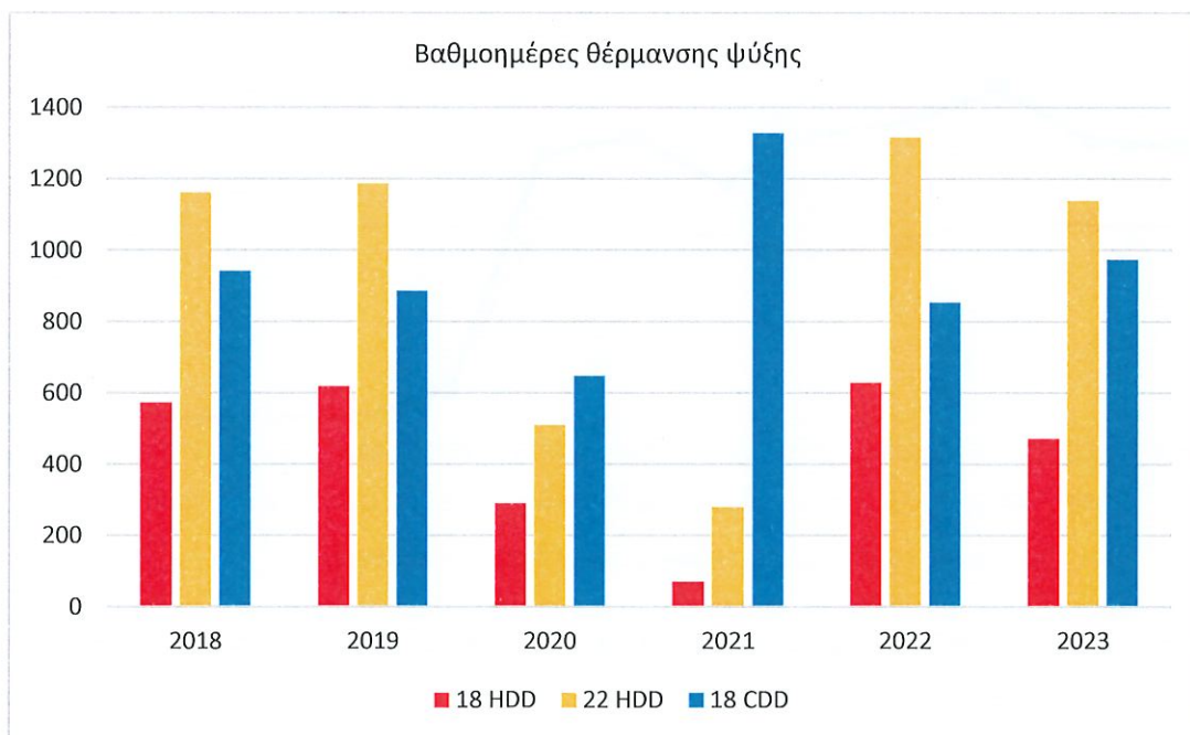
Σχήμα 12: Βαθμομέρες θέρμανσης (αριστερός άξονας) και ψύξης (δεξιός άξονας) για την περίοδο 2018-2023.
