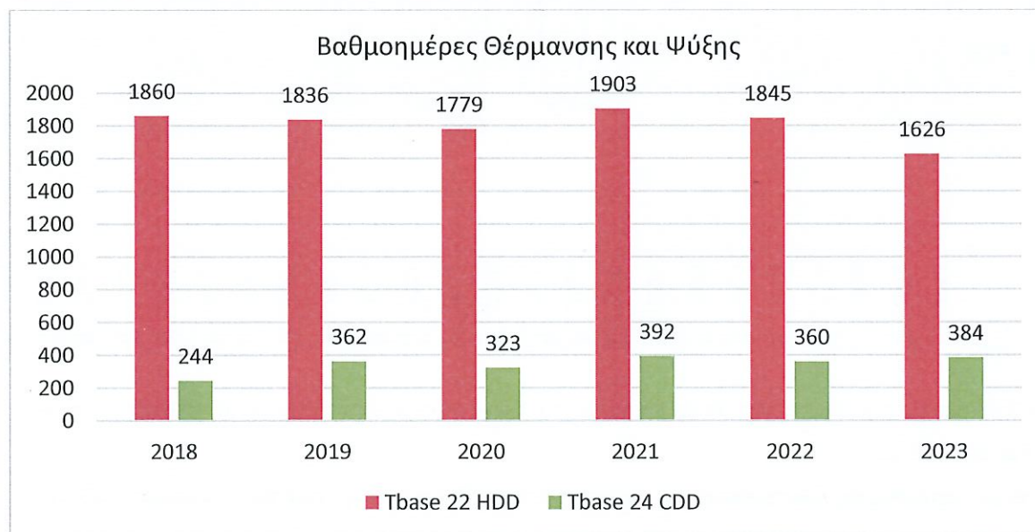
Σχήμα 7: Βαθμομέρες θέρμανσης (hdd με θερμοκρασία βάσης 22 οC) και ψύξης (cdd με θερμοκρασία βάσης 24 οC) για την περίοδο 2018-2023 στο ΜΠΚ
